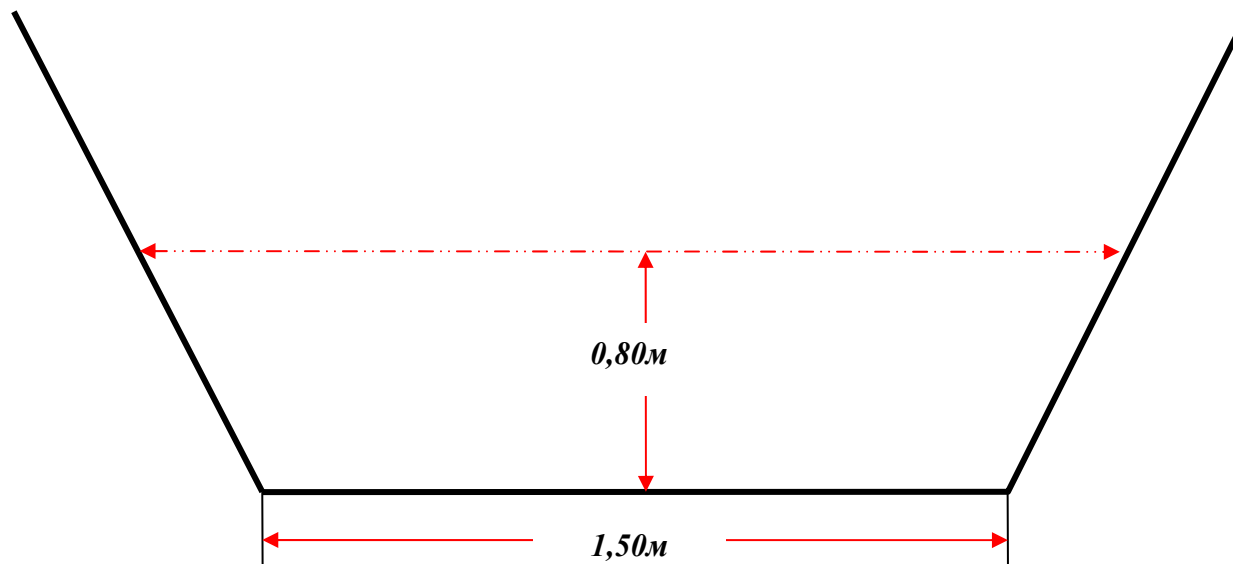
Прилог бр. 6. – Карактеристичан попречни профил корита канала тзв. “Брза вода “ у КО Бунушки Чифлук-Д.Бунуша до улива у канал Ботуњу
