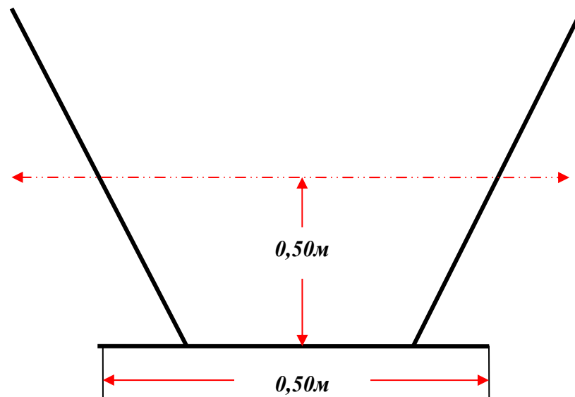
Прилог бр. 10. – Карактеристичан попречни профил корита одводног канала из села до канала Ботуња у КО Радоњица
