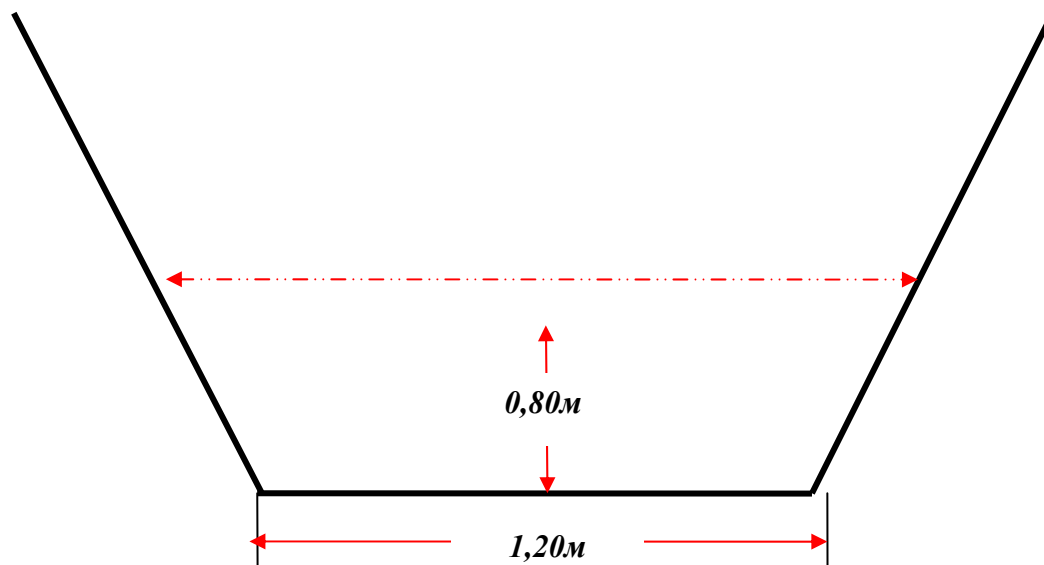
Прилог бр. 9. – Карактеристичан попречни профил корита канала тзв. „Барски канал“ у КО Радоњица-КО Стројковце
